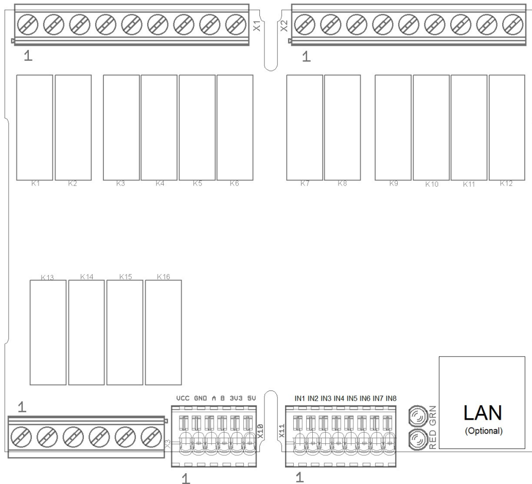
Ansicht von Oben: Stecker und Klemmenposition
